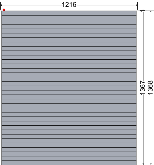
Innen Ansicht
