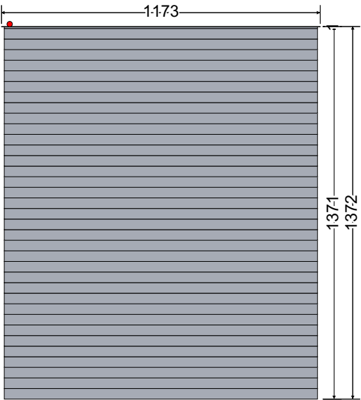
Innen Ansicht
