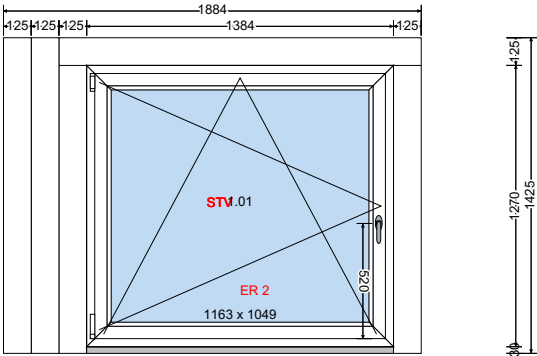
Innen Ansicht
