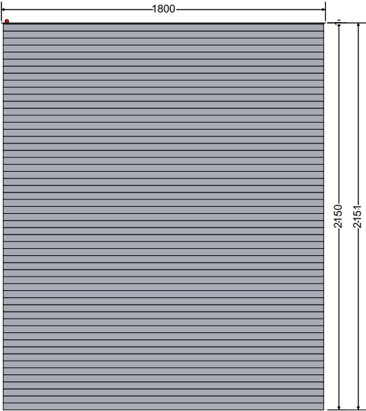
Innen Ansicht
