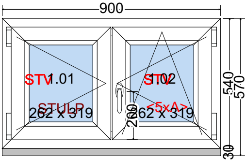
Innen Ansicht
