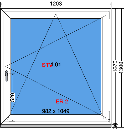
Innen Ansicht
