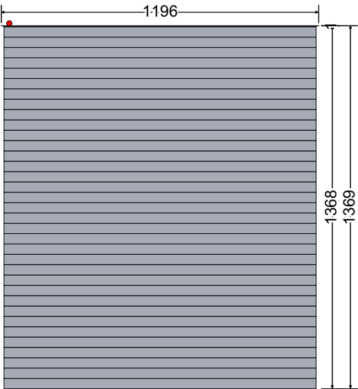
Innen Ansicht
