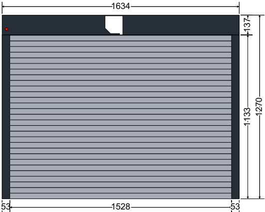
Innen Ansicht
