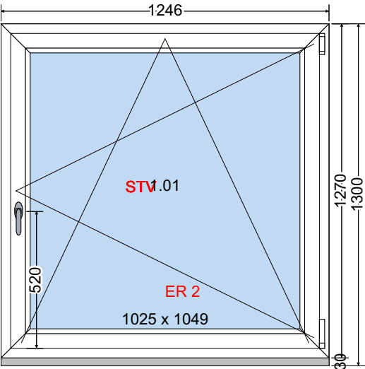
Innen Ansicht
