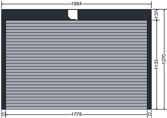
Innen Ansicht
