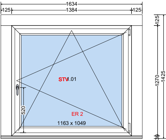
Innen Ansicht
