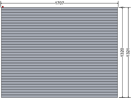
Innen Ansicht
