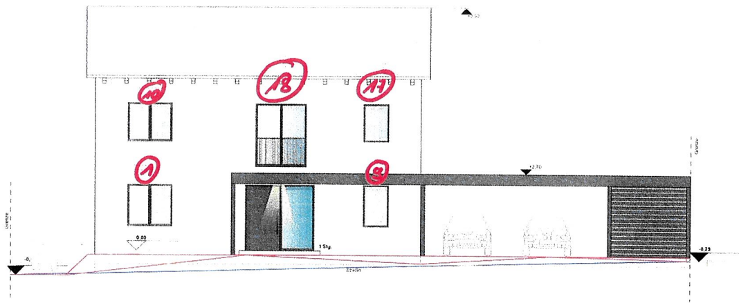
Ansicht Norden
